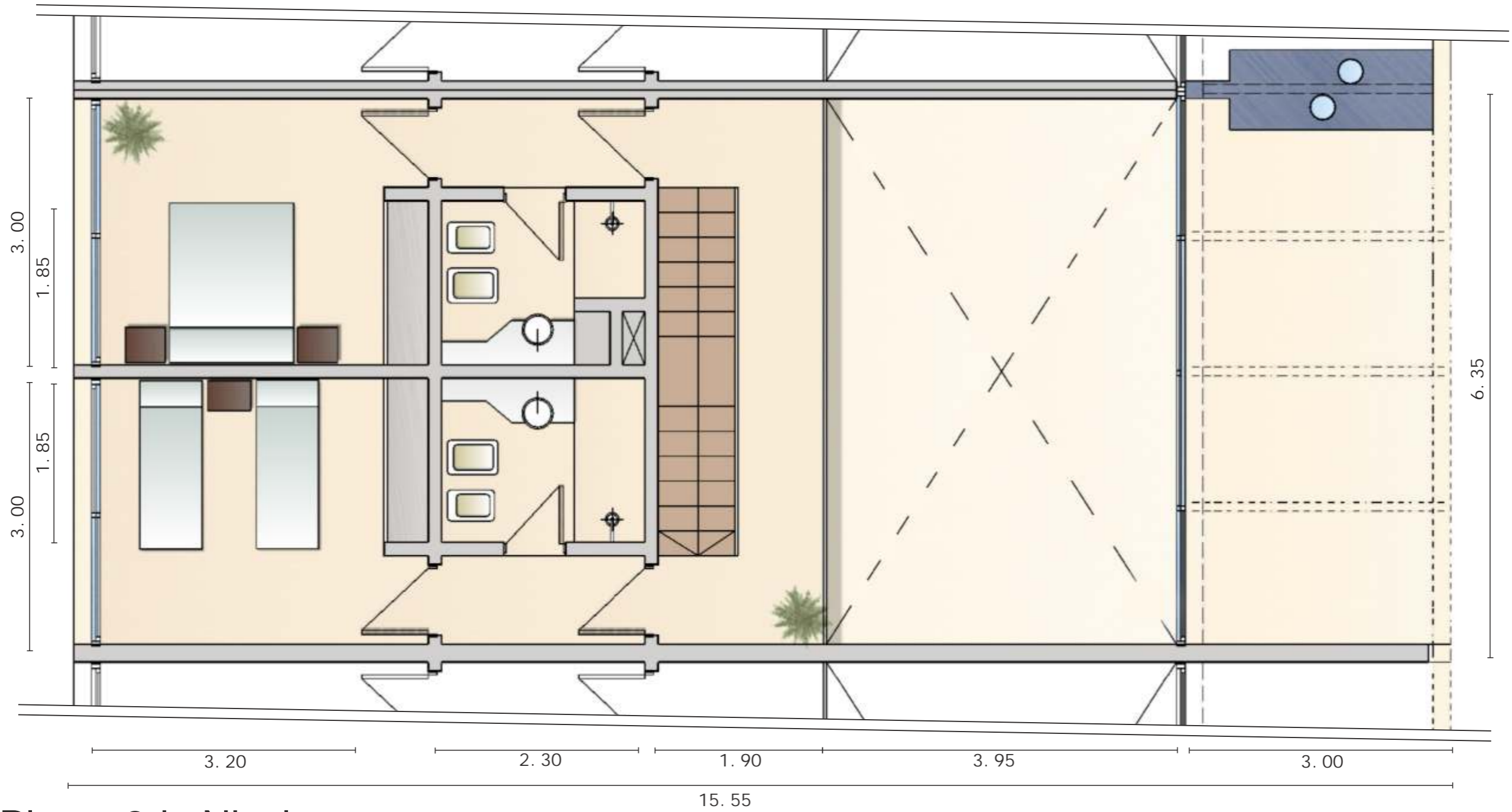
Planta 2do Nivel
